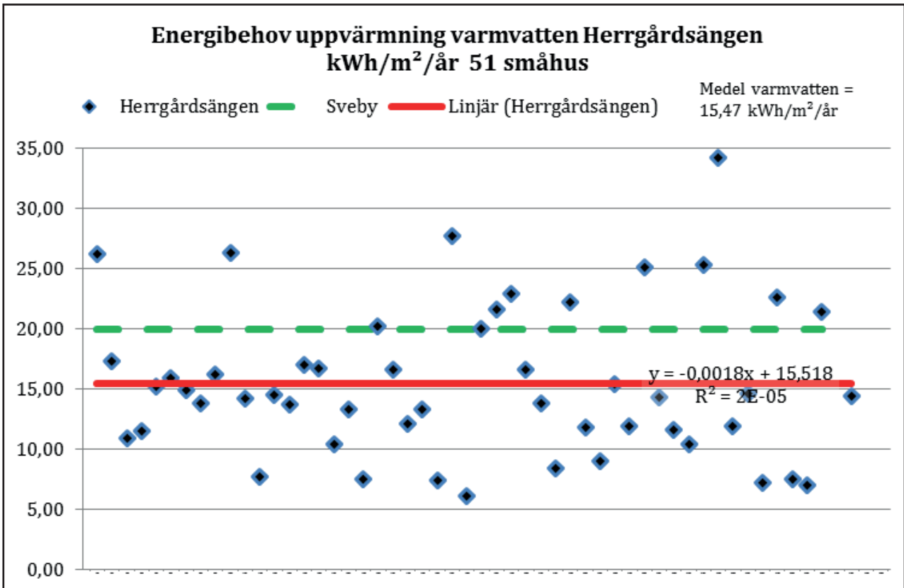
Figur 6.10 Sveby = Brukarindata för bostäder småhus årsschablon Svebyprogrammet version 1.0 2012-10-10
